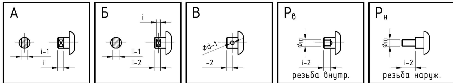
Рис.1. Вариант исполнения оси А, Б, В, Pв, Pн
